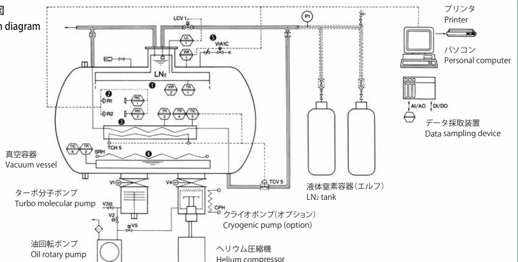
小型スペースチェンバー系統図
